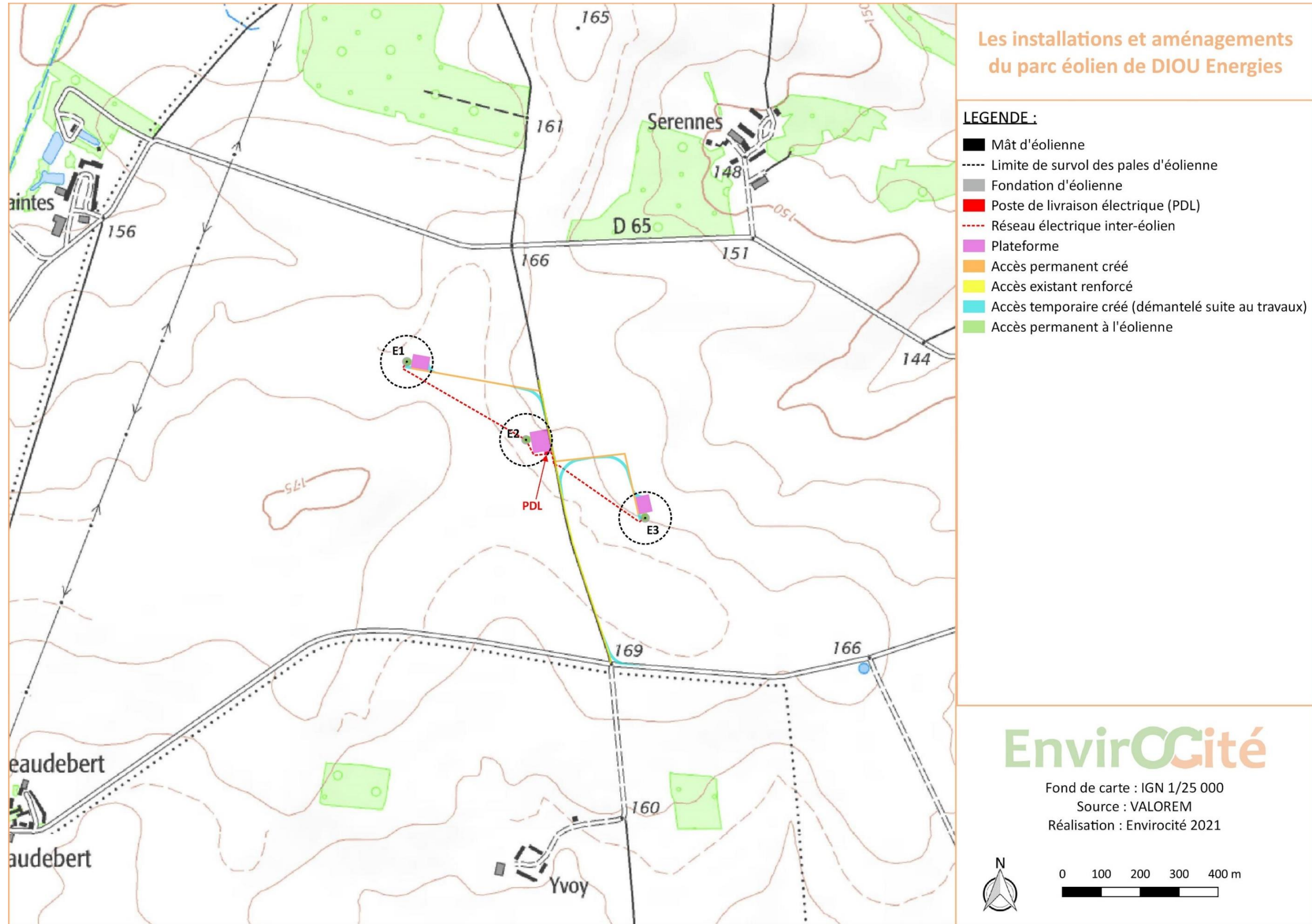
Carte 6 : Localisation des installations et aménagements du projet de parc éolien sur fond scan 25
