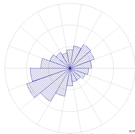
Figure 1 : rose des vents du site (Source : VALOREM)
