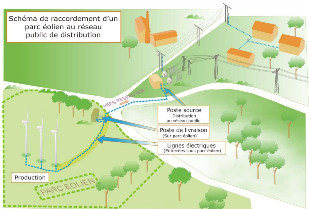
Figure 4 : Schéma de la structure de raccordement au réseau public de distribution (Source : ADEME)
