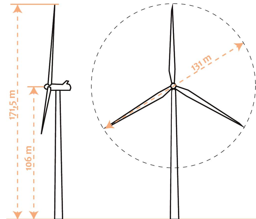
Figure 5 : Gabarit maximum de l'éolienne retenue
